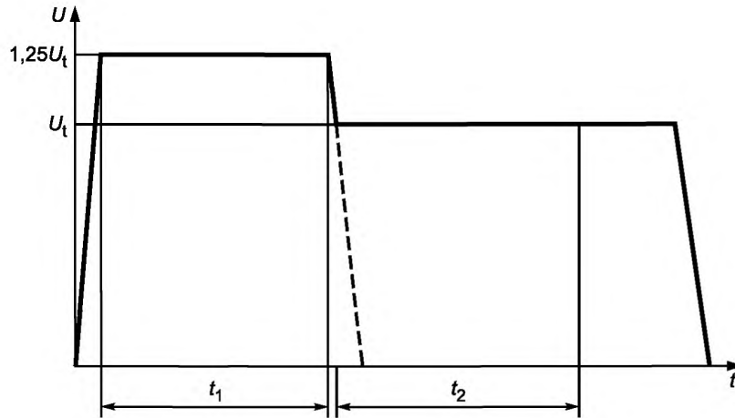
Рисунок 3 – Испытательное напряжение
