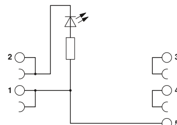
Схема подключения PLC-VT/ACT/LA
