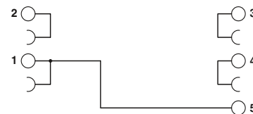
Схема подключения PLC-VT/ACT
