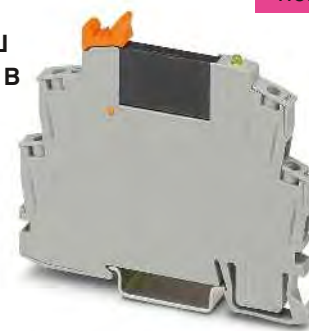
Модуль полупроводникового реле с винтовыми зажимами, выход пост. тока макс. 3 А
