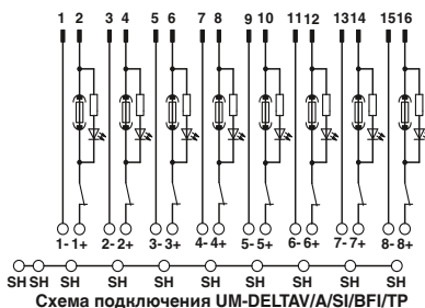
Схема подключения UM-DELTA V/A/SI/BFI/TP
