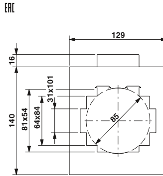
Шинный трансформатор тока заказчик может выбрать калибруемый вариант
