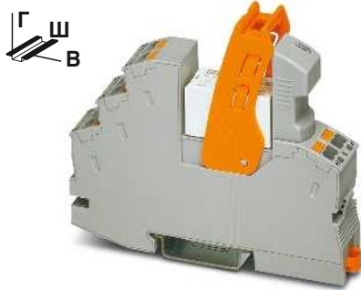
Релейный модуль с 2 переключающими контактами с Зажим push-in
