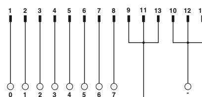
Схема подключения VIP-2/.../FLK14/8P/PLC
