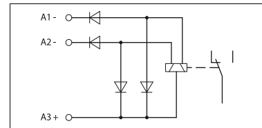
Принципиальная схема бистабильного реле с отрицательной полярностью
