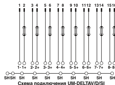
Схема подключения UM-DELTA V/D/SI
