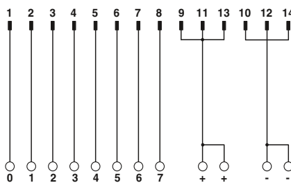
Схема подключения VIP-2/.../FLK14/LED/PLC
