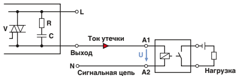
Возникновение паразитных сигналов: Вариант 1: управление - выходная плата переменного тока
