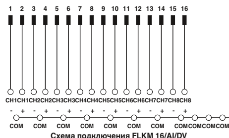
Схема подключения FLKM 16/AI/DV
