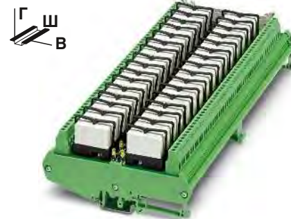
Модуль вывода с 32 миниатюрными реле, 1 переключающий контакт
