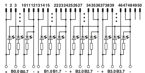
Схема подключения VIP-2/.../FLK50/LED/PLC
