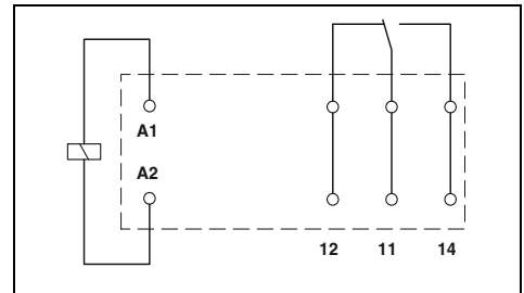
Реле с 1 переключающим контактом для повышенного тока длительной нагрузки, макс. 16 А
