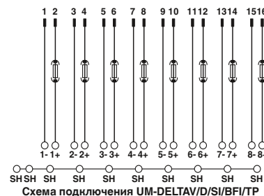
Схема подключения UM-DELTA V/D/SI/BFI/TP
