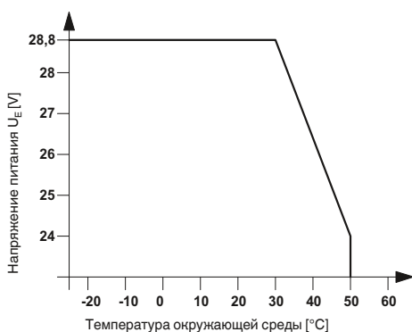
Изменение характеристик для EIK 1-SVN 24 P
