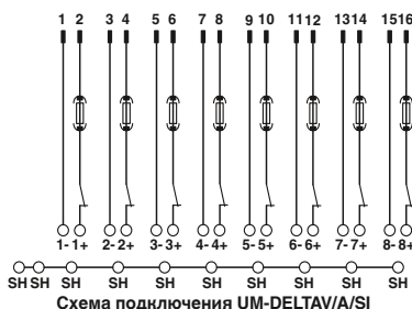
Схема подключения UM-DELTA V/A/SI
