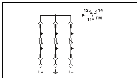
Штекерное устройство защиты от перенапряжения и тока молнии для ФГ-приложений до 1000 В пост. тока
