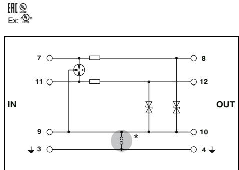
2 проводника, с общим опорным потенциалом, например, для двоичных сигналов
