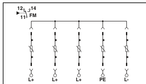
Вставное устройство защиты от перенапряжений, для ФГ-приложений до 1000 В пост. тока, 3 устройства слежения MPP
