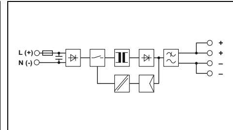
Источник питания, 1-фазный, 12 В DC, 1,5 А плоская конструкция, NEC, класс 2
