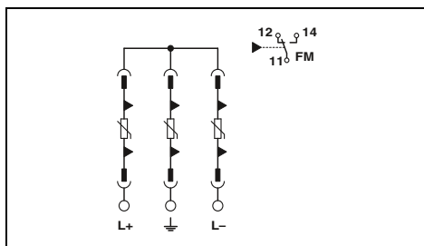
Вставное устройство защиты от перенапряжений, для ФГ-приложений до 1000 В пост. тока, 1 устройство слежения MPP
