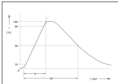
Импульс тока формы 8/20 согласно МЭК 60060-1
