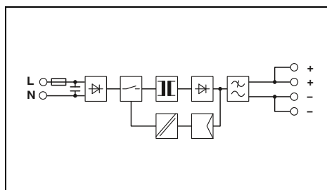
Источник питания, 1-фазный, 48 В DC, 60 Вт
