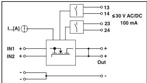
Активный модуль резервирования, с защитным покрытием 24 В DC, 2x 10 А, 1x 20 А ClassNK
