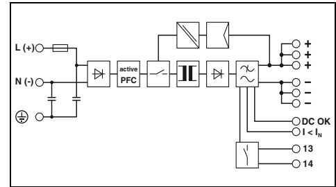
Источник питания, с защитным покрытием, 1-фазный, 24 В DC, 5 А
