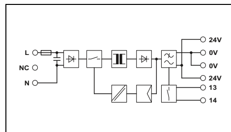
Источник питания, 1-фазный, 24 В DC, 1,5 А, Опциональные шинные соединители для DIN-рейки
