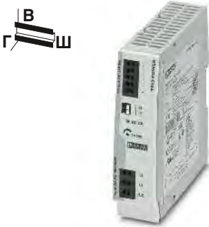
Источник питания, 3-фазный, 24 В DC, 5 А
