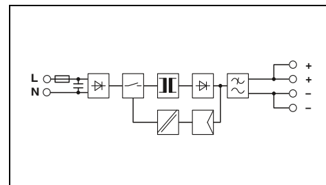
Источник питания, 1-фазный, 24 В DC, 60 Вт NEC, класс 2
