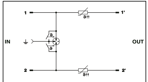
2-линии, грубая защита, с отагоустойчивым контактом и токовой защитой (Powercross)
