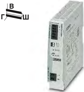
Источник питания, 1-фазный, 24 В DC, 3 А, NEC Class 2
