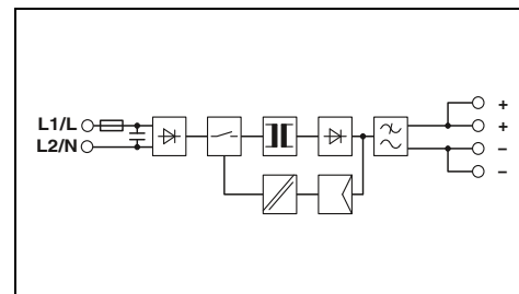
Источник питания, 2-фазный, 24 В DC, 90 Вт NEC, класс 2
