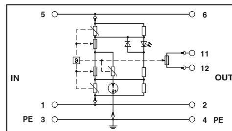
Для источников питания 230 В перем. тока, 3-проводная система, L1, L2, PE (системы ИТ)
