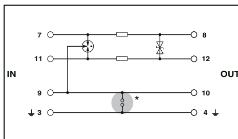
Двойная жила (петля), без потенциала земли, например, для токовых контуров 4 ... 20 мА
