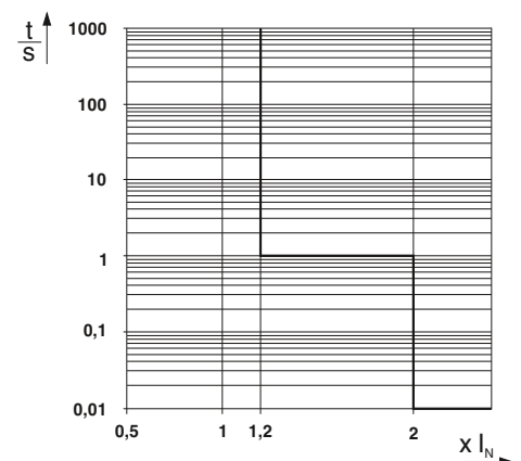
Характеристика срабатывания в диапазоне постоянного тока
