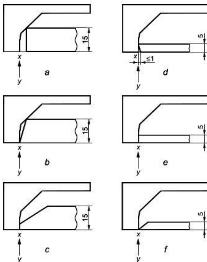
Рисунок 104 - Пример применения калибра согласно рисунку 102 в соответствии с 11.102.7
