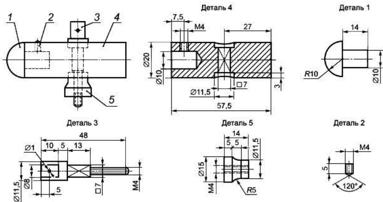
Рисунок 108 - Ударный элемент установки
