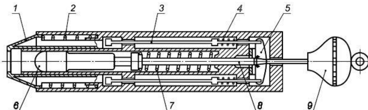
Рисунок 112 - Прибор для испытания ударом
