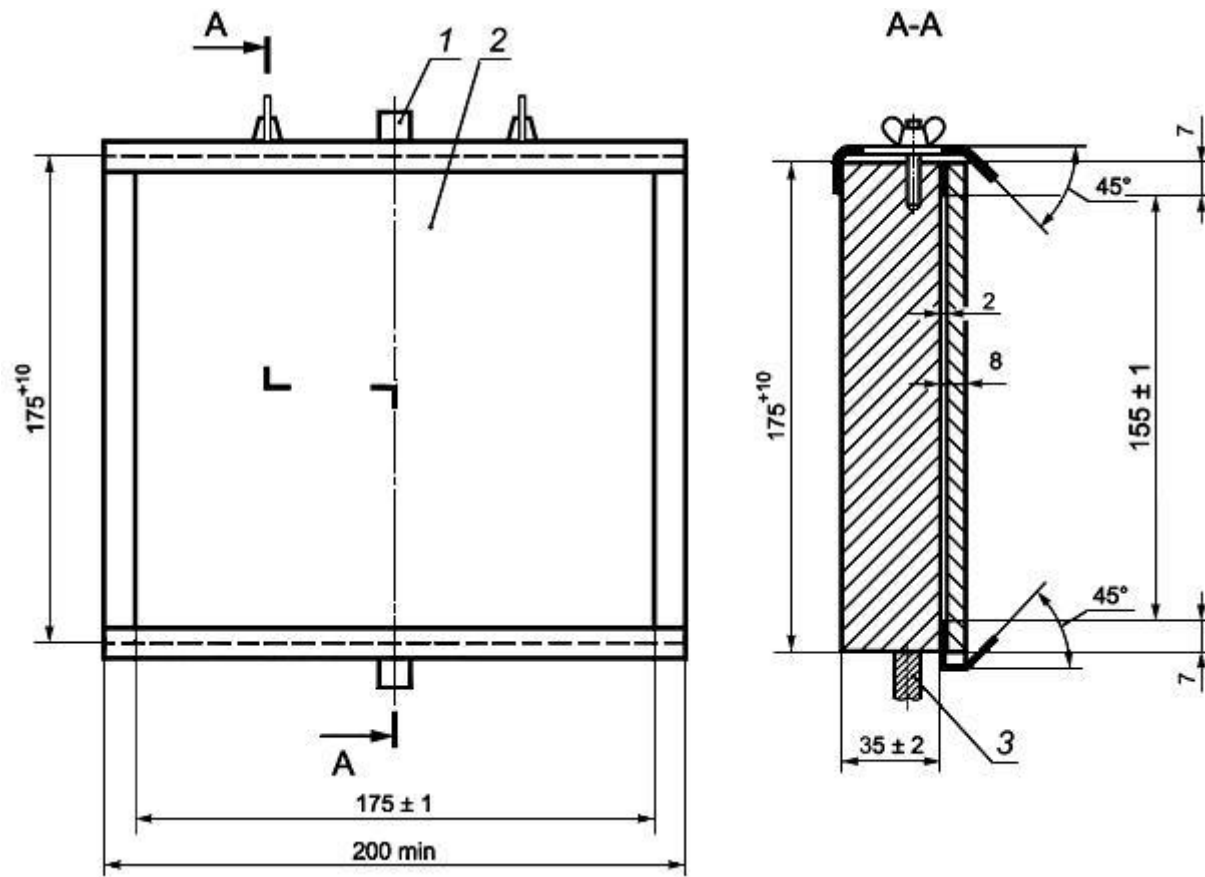
Рисунок 109 - Монтажная опора для образцов
