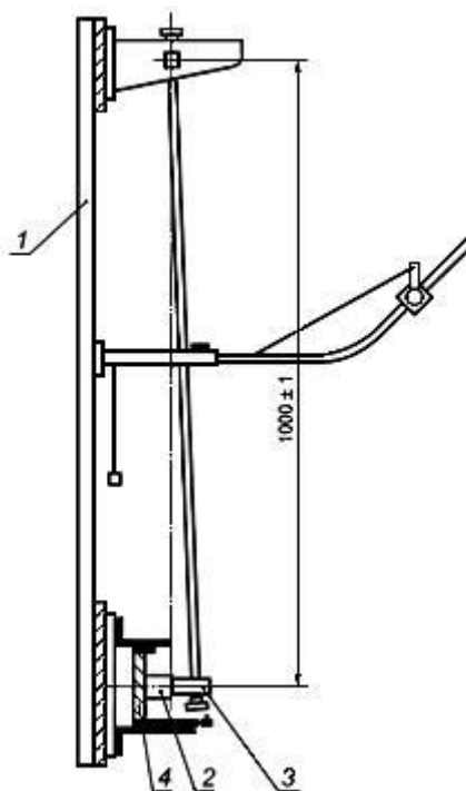
Рисунок 107 - Установка для проверки механической прочности образцов
