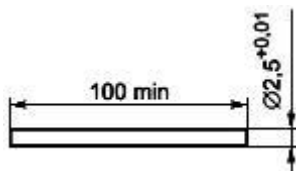
Рисунок 105 - Калибр (в виде металлического стержня) для проверки пазов, отверстий и обратных конусов
