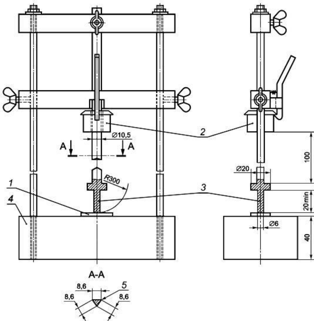
Рисунок 111 - Установка для испытания ударом при низкой температуре
