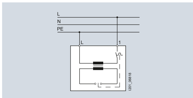
Розетка для бритья (принципиальная электросхема)
