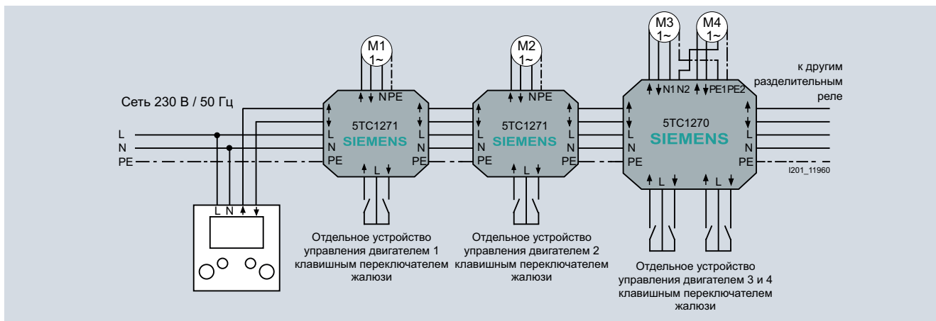
Схема соединения
